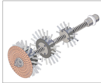
Twister (ungelinerte)
