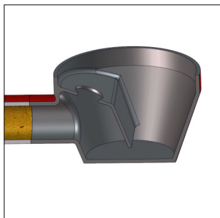
BODENABLAUF
