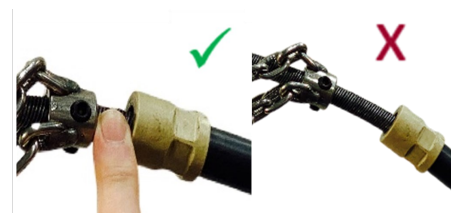
Achten Sie darauf, dass der Abstand zwischen Endkappe und Werkzeug ca. 6mm beträgt (fingerbreit).
