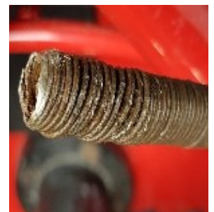
Zurückschneiden beschädigter Welle
